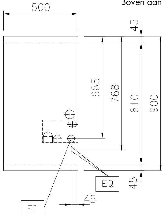
Boven aanzicht
